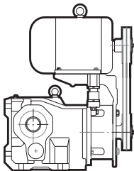
Bevel Unit
